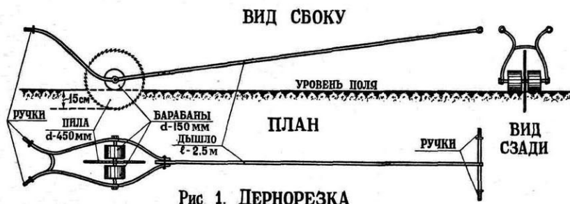
Рис 1. ДЕРНОРЕЗКА
